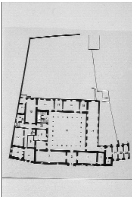
Lámina 3: Planta baixa do Colexio de Santiago Alfeo, segundo Fraguas.
